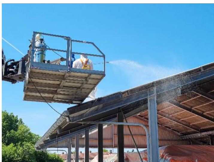
Foto 28: Inschuimen nokstukken (zijkant)
