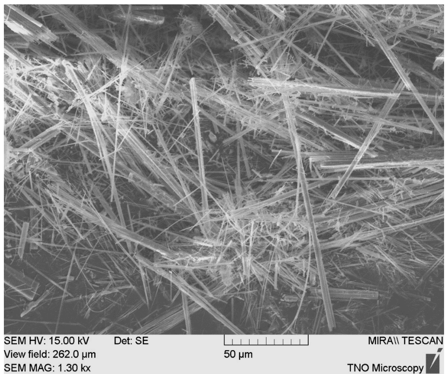
Foto B5-2: Voorbeelden van amosietvezels aangetroffen in preparaat van materiaalmonster (SEM/RMA)
